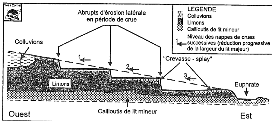
Fig.8. - Profil transversal schématique dans la plaine alluviale de l'Euphrate (rive droite) à Jerablus; illustration de la réduction progressive de la largeur du lit majeur de l'Euphrate.
