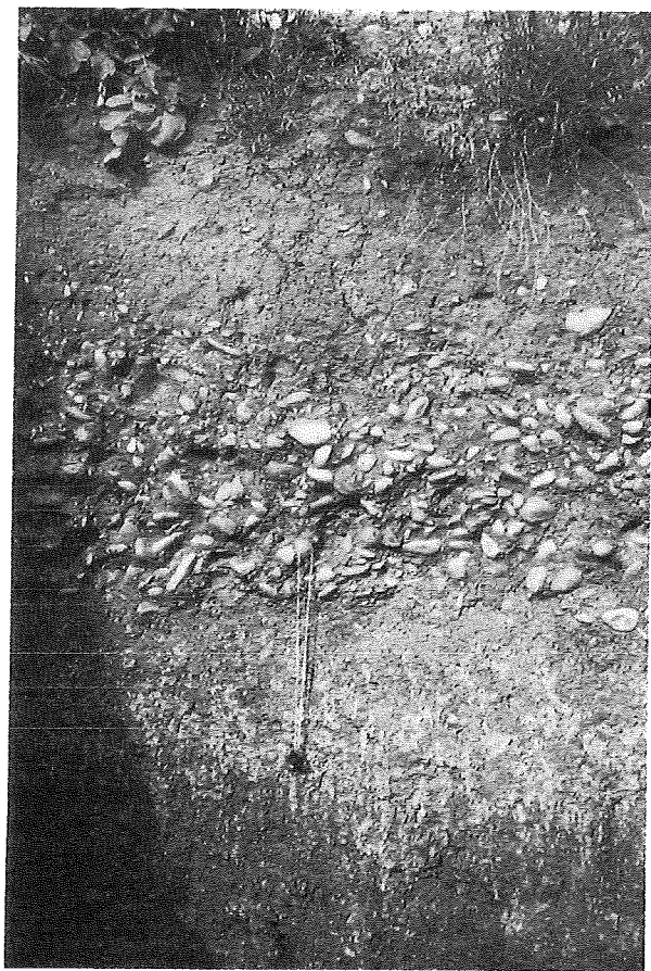
Fig.7. - Dépôt de type crevasse - splay entre Jerablus et Jerablus Takhtani .
