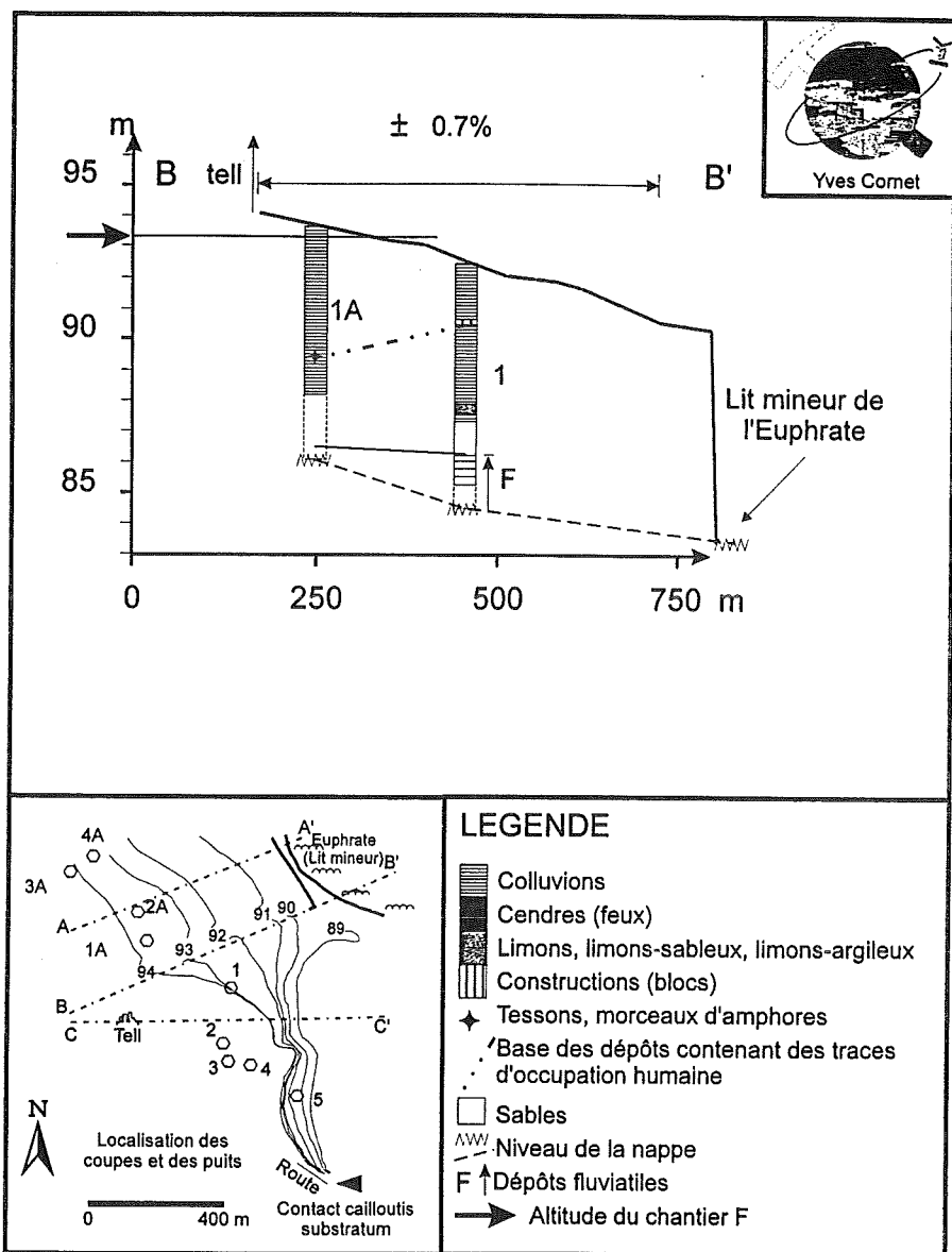
Fig. 6. - Synthèse des observations réalisées dans les puits d'Amarna et reportées par projection à altitude constante sur 3 coupes topographiques traversant le cône de déjection du wadi Amarna (Localisation précise sur la figure 2).
